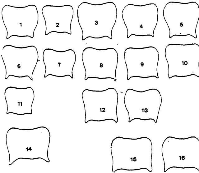
Abb. 1. Halsschildumriß.
